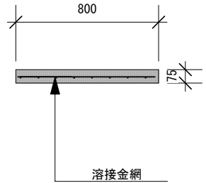
土間コンクリート標準構造図 S=1:25
